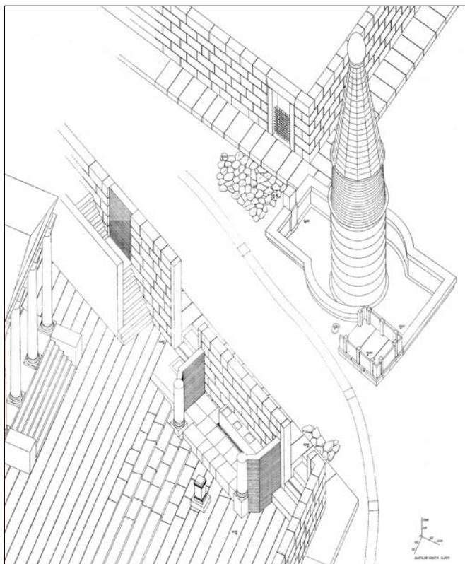
Fig. 31. Assonometria ricostruttiva dell'area in età claudia (dis. dell'A.).
