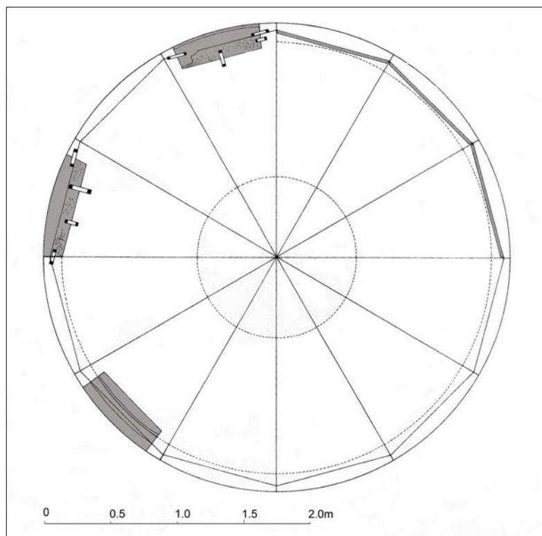
Fig. 25. Fontana di età augustea. Sezione orizzontale ricostruttiva del saliente all'altezza della seconda cornice, con il posizionamento dei blocchi ritrovati e delle lastre di rivestimento della cuspid (dis. dell'A.).
