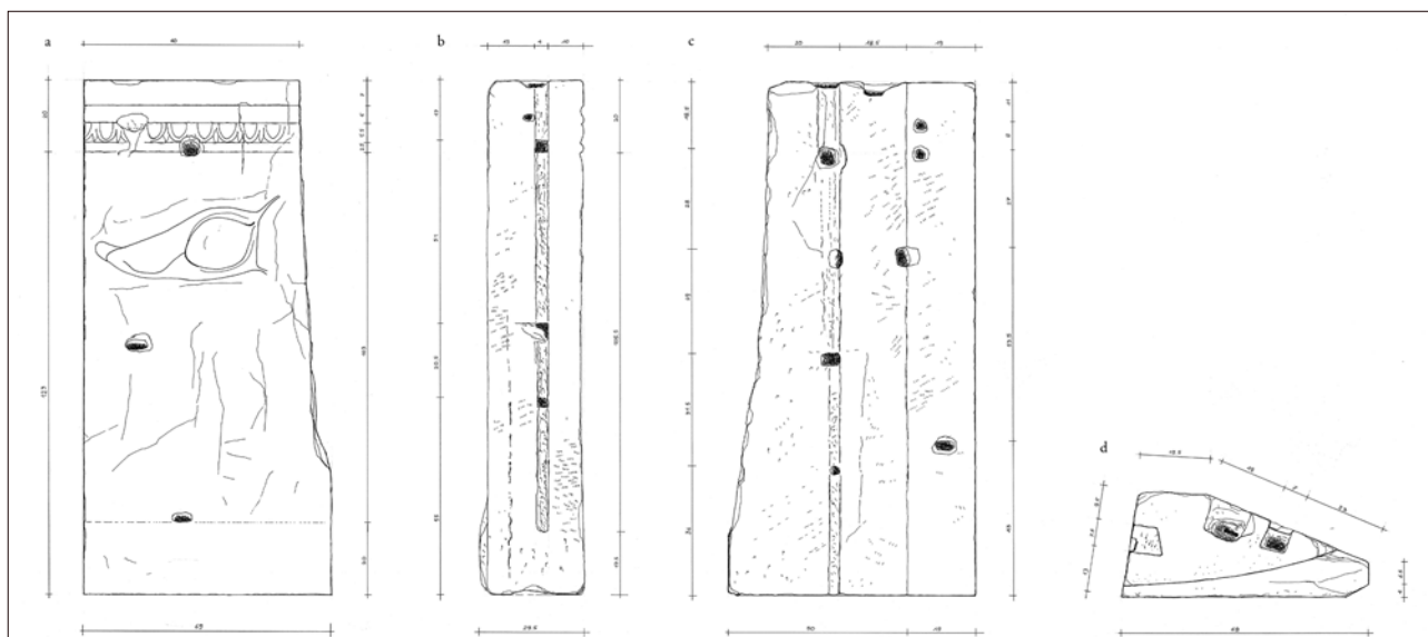
Fig. 24. Rilievo della lastra del parapetto augusteo riusata come tombino nel rifacimento claudio: a) fronte, b) faccia laterale di contatto; c) retro; d) pianta del letto di attesa (ril. dell'A.).
