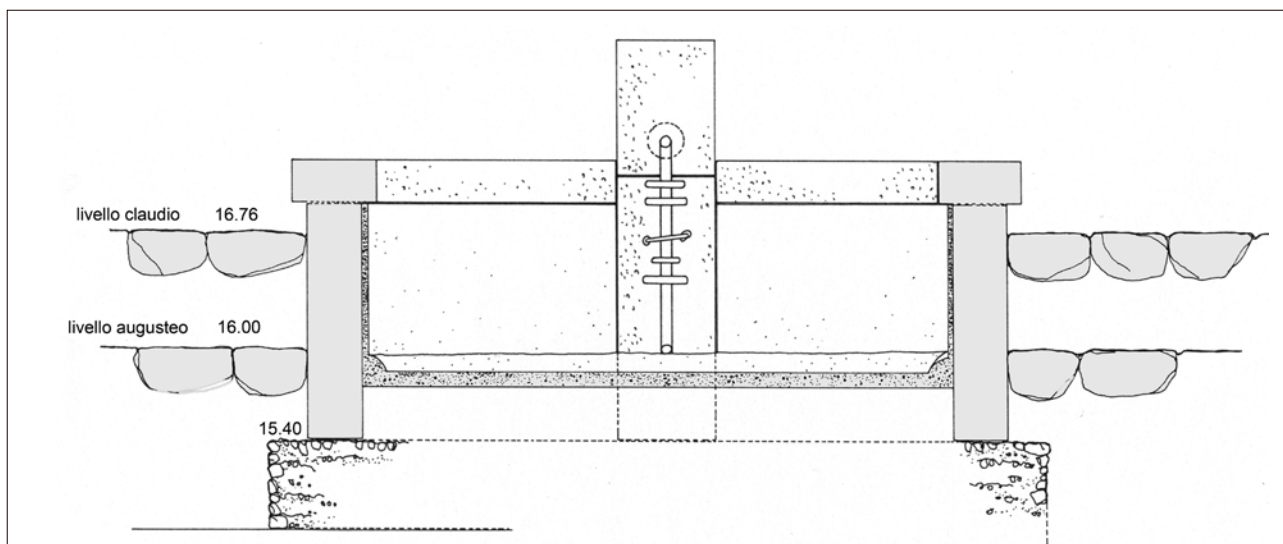
Fig. 8. Roma, meta augustea. Parapetto occidentale della vasca, prospetto interno, sul quale era fissata una fistula in piombo che alimentava una fontanella (dis. dell'A.).
