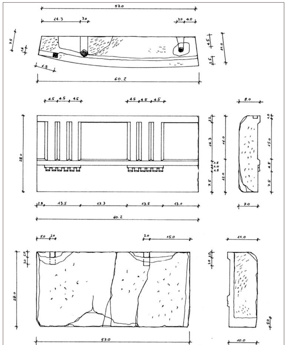
Fig. 16. Rilievo della trabeazione di ordine dorico, inv. 2703 (dis. dell'A.).
