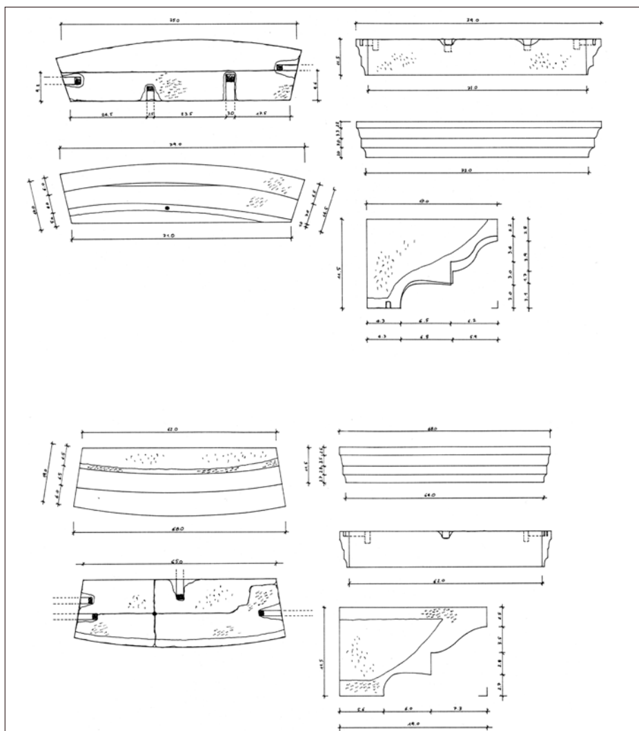
Fig. 17. Rilievo delle cornici del secondo livello, inv. 2486 e 2487a-b (dis. dell'A.).
