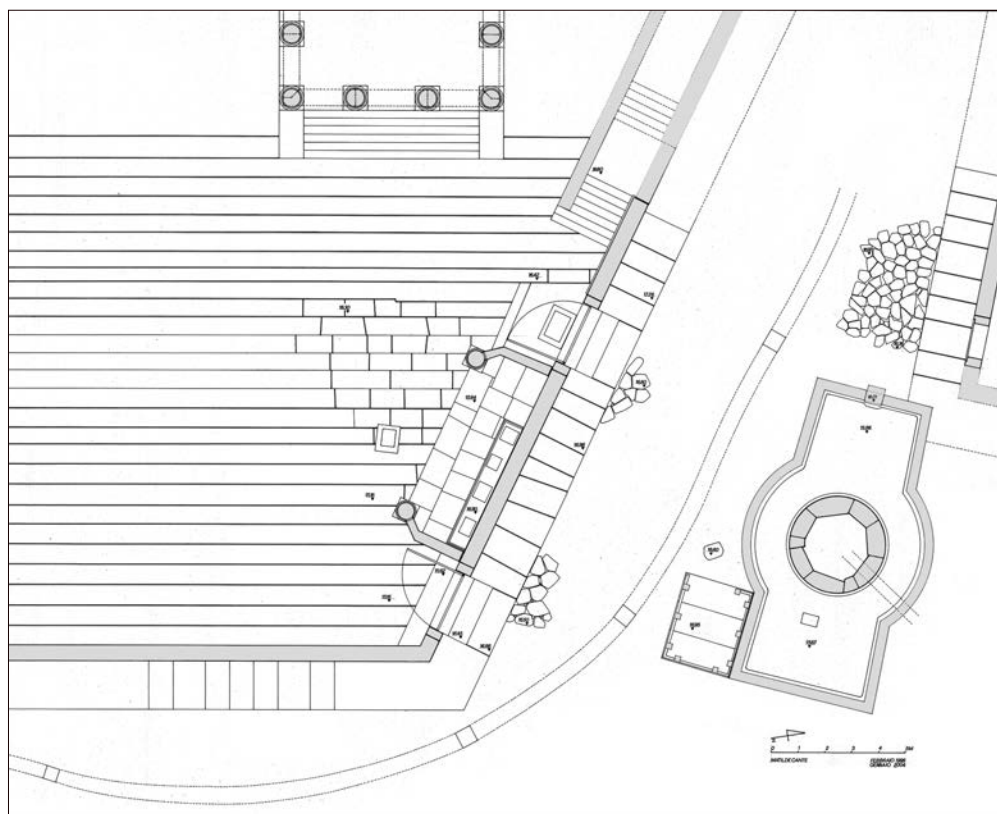
Fig. 3. Roma. Planimetria ricostruttiva del complesso meta-compitum e del santuario delle Curiae Veteres nella fase di età claudia, 51-54 d.C. (dis. dell'A.).
