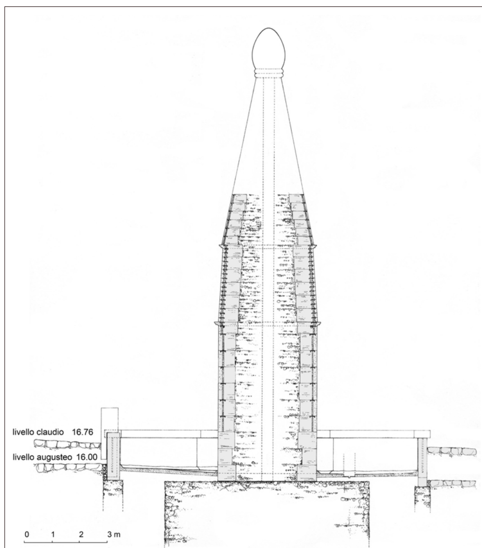
Fig. 29. Fontana di età augustea. Ipotesi di restituzione della sezione longitudinale (dis. dell'A.).
