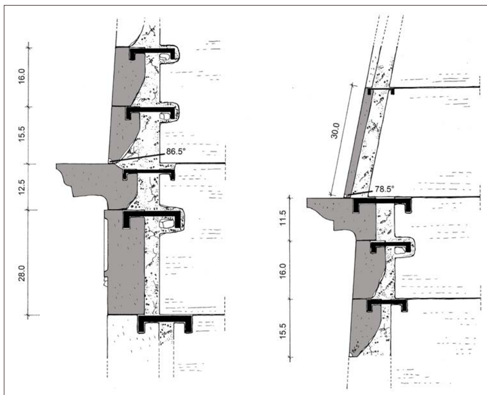
Fig. 28. Fontana di età augustea. Particolari costruttivi: sezione del montaggio delle cornici del primo e del secondo livello (dis. dell'A.).
