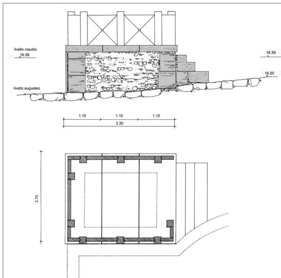
Fig. 30. Ipotesi di restituzione del compitum , sezione e pianta (dis. dell'A.).
