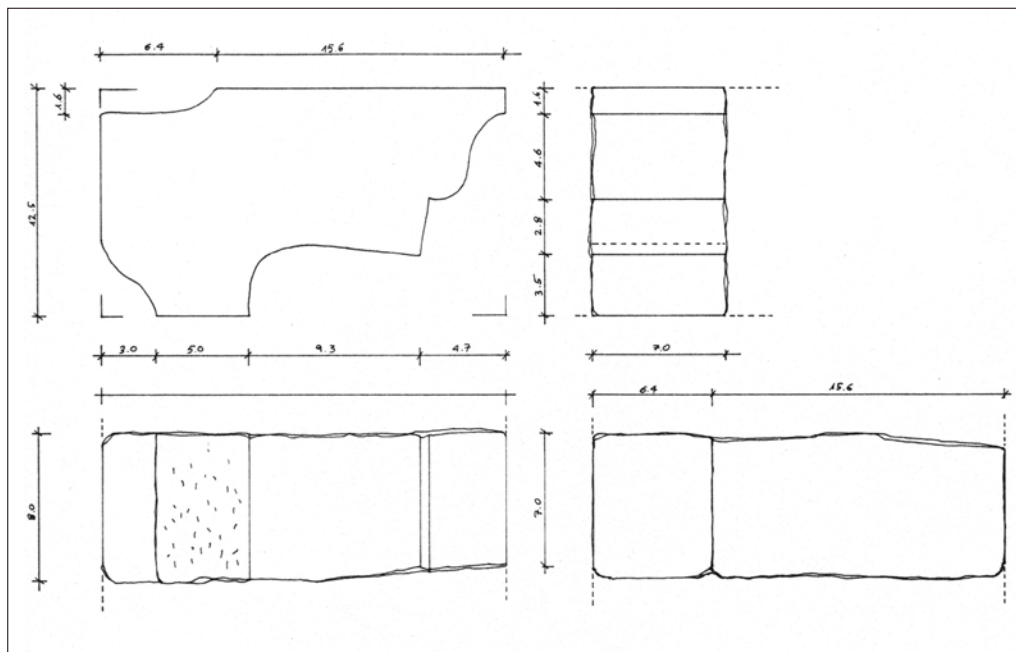
Fig. 19. Rilievo del frammento della cornice del primo livello, inv. 2702 (dis. dell'A.).
