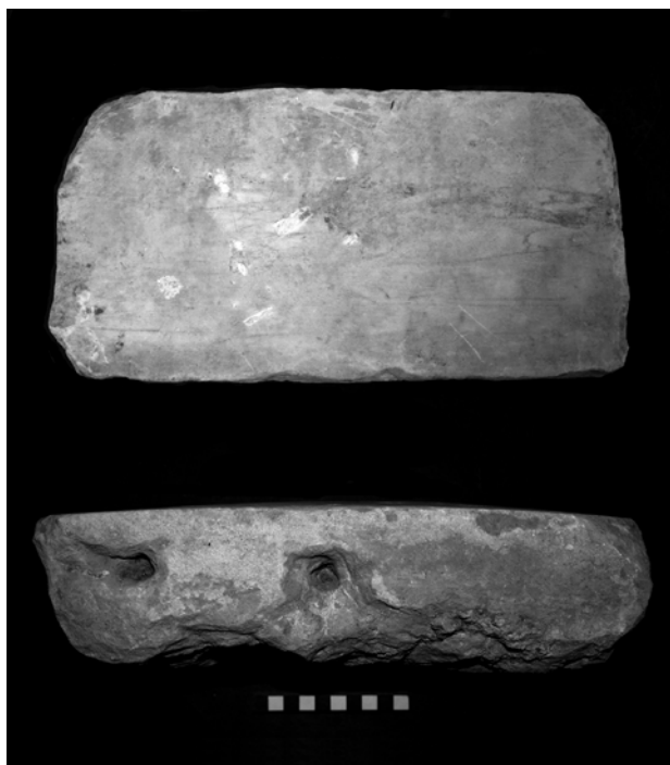
Fig. 21. Blocco curvilineo di opera isodoma appartenente al settore troncoconico del saliente, inv. 2704 (foto G. Pardini).
