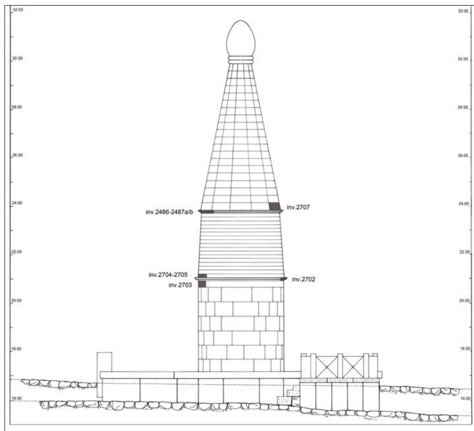
Fig. 27. Fontana di età augustea. Ipotesi di ricostruzione: del prospetto laterale con indicazione dei frammenti identificati (dis. dell'A.).
